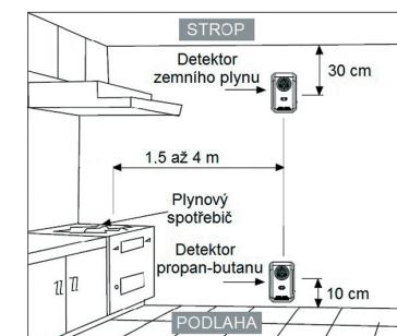
Umístění detektorů hořlavých plynů.
