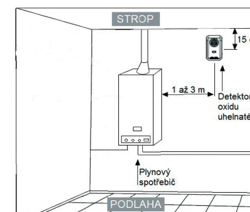
Umístění detektorů oxidu uhelnatého.
